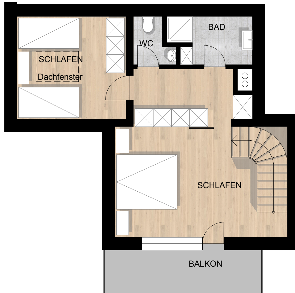
Obergeschoss
